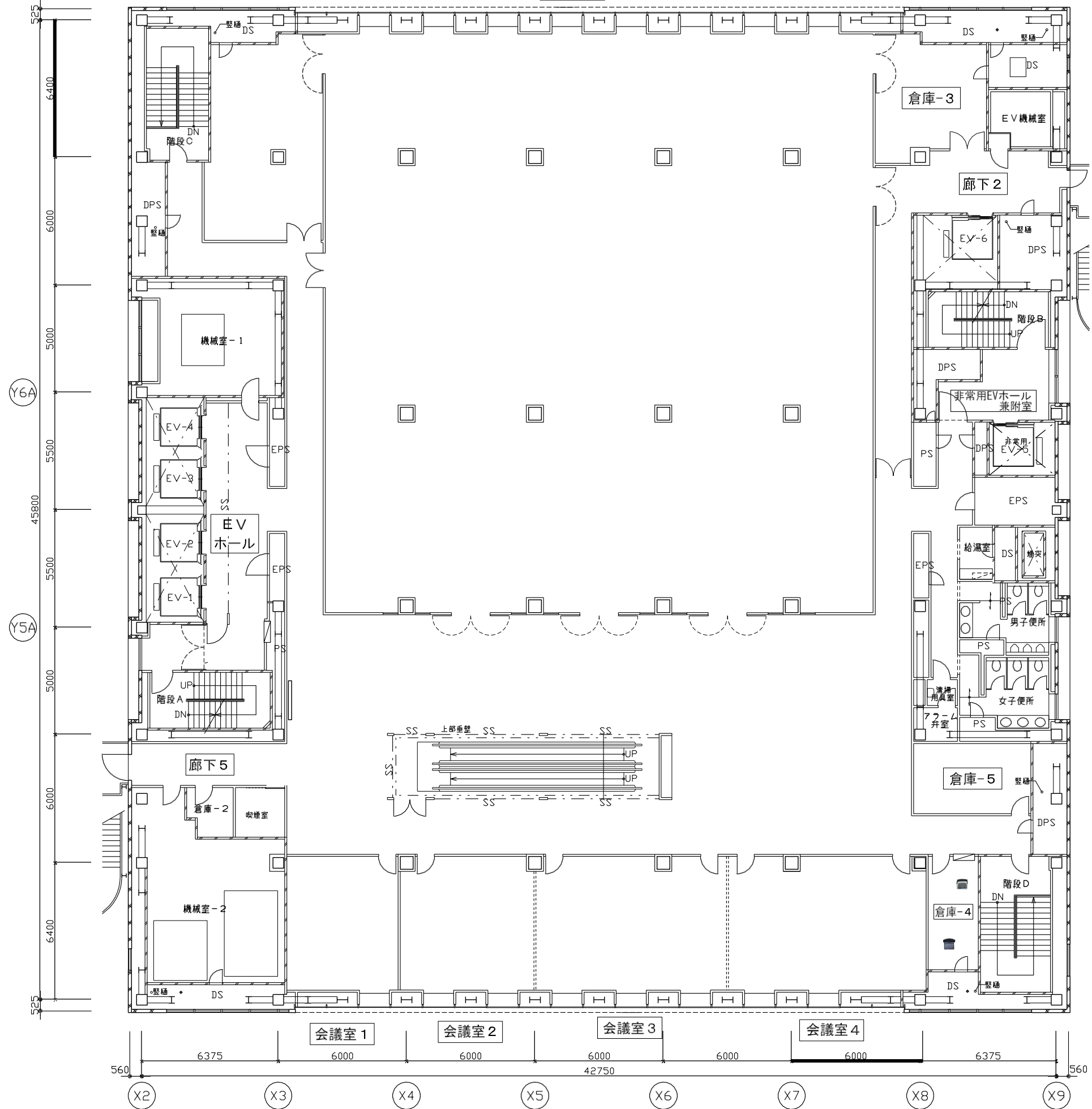
3階平面図 1/100
